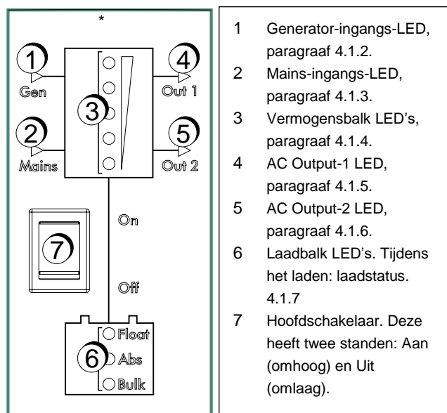
Afbeelding 4-1: Frontpaneel
