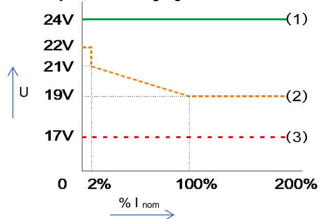
Afbeelding 4-2: Dynamisch DC-ingangsvenster
